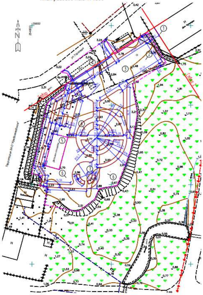
План разбивочный М 1:500
